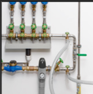
Ispiranje instalacija pitke vode vodom ili mešavinom vode i vazduha 1)(3)(4)
