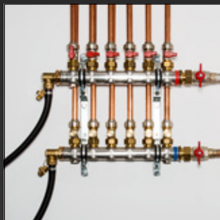
Odmuljavanje i ispiranje sistema grejanja. 2)
