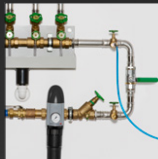
Ispitivanje pod pritiskom uz pomoć komprimovanog vazduha (SL / SLW) 4)(7) Ispitivanje pod pritiskom uz pomoć vode (SLW) 1)(6)
