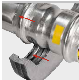
Örnek REMS Presleme pensleri Mini V: Fittinglere preslenmiş geriye dönüp takip etmek için "V" baskısı EN 1775:2007'e uygun.
