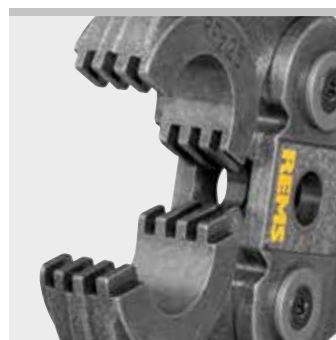
Užspaudimo replės su dantukais apsaugo nuo išlajų susidarymo prie presuojamosios jungties Patentas EP 2 027 971
