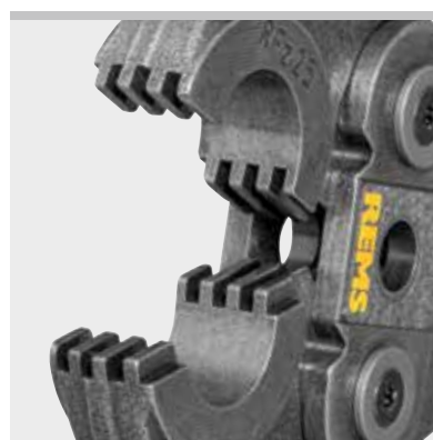
Les pincès à sertir sont munies d'une denture pour prévenir la formation de bavures sur le raccord à sertir. Brevet EP 2 027 971
