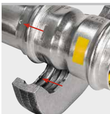
Exemple pince à sertir Mini REMS de profil V: Marquage „V” sur le raccord sertí permettant la traçabilité selon norme EN 1775:2007
