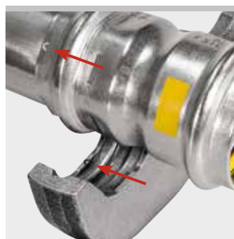
Příklad lisovacích kleští REMS Mini V: Otisk "V" na zatísované tvarovce pro zpětné dosledování dle EN 1775:2007
